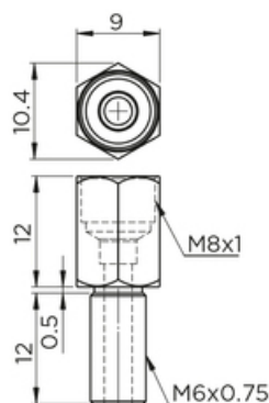
OA-M6-M8-L
